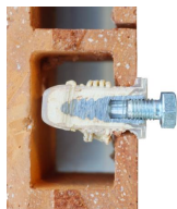
Insert taraudé - vue en coupe
