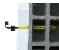
Arrêt de volet ISO - vue en coupe
