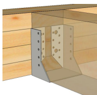
Sabot de charpente à ailes intérieures - en situation
