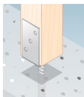
Pied de poteau en U à ancrer - vue en situation
