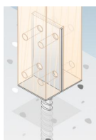
Pied de poteau en âme à ancrer - vue en situation
