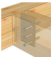
Broche connecteur - vue en situation
