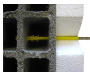
Fixation pour accessoire ISO - vue en coupe
