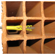
Cheville traversante - vue en coupe dans la brique rouge
