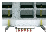
Cheville chaudière murale avec doublage - vue en coupe
