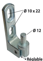
Pivot de portail PVC - côtes
