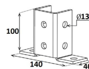
Equerre 3 faces 90° - schéma technique
