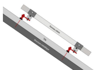
Fixation solaire filet métrique - schéma
