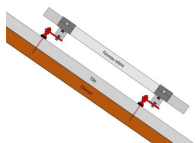
Fixation solaire - schéma
