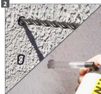
2 Percez Ø 20 mm puis nettoyez le trou à l'aide d'une pompe soufflante
