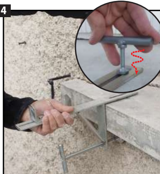
4 Visser manuellement la rallonge sur l'appui de fenêtre à l'aide de la clé.
