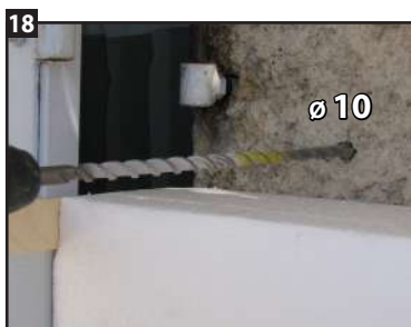
18 Percer un trou Ø10 mm au centre du repère.
