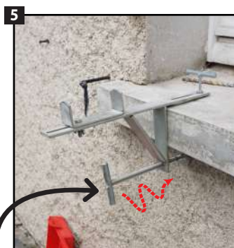
5 Serrer la pièce contre le crépi pour faire contrepoinds.
