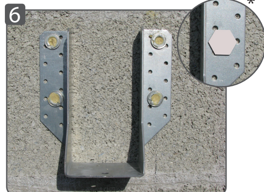
6 Le sabot de charpente est fixé. Mettre les capuchons de recouvrement pour l'esthétique (facultatif). *
