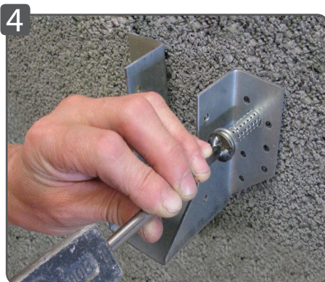
4 Frapper le 1er clou à travers le sabot de charpente à l'aide de l'outil de pose.
