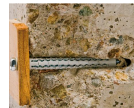
Cheville CQLV Ø8 - vue en coupe dans le béton
