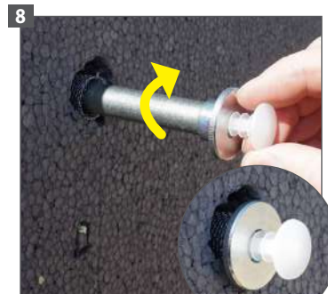
Vissez et enfoncez en même temps la fixation.
