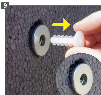
Une fois la résine durcie, retirez le bouchon de protection.
