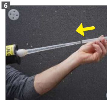
Placez la rallonge sur l'embout mélangeur et faites monter la résine jusqu'au bout.
