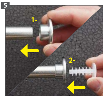
Anticipez en enfonceant la rondelle d'appui et le bouchon de protection dans le taraudage.
