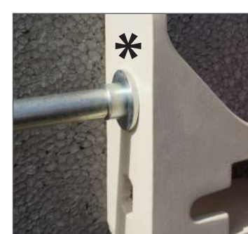
La rondelle d'appui est en place derrière le support pour éviter l'écrasement.
