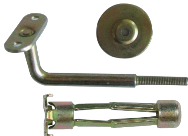
Fixation main courante M8 plaque de plâtre
