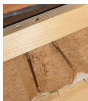
Vis toiture - vue en coupe
