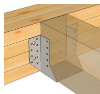
Sabot de charpente à ailes extérieures - en situation
