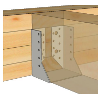
Sabot de charpente à ailes intérieures - en situation
