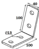
Equerre d'assemblage 4 trous 90° - schéma technique
