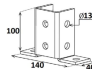
Equerre 3 faces 90° - schéma technique
