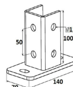
Pied profil acier lourd - schéma technique
