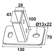
Pied profil acier léger - schéma technique
