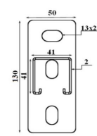
Console 41 x 41 - schéma technique
