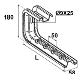
Equerre universelle CWU - schéma technique
