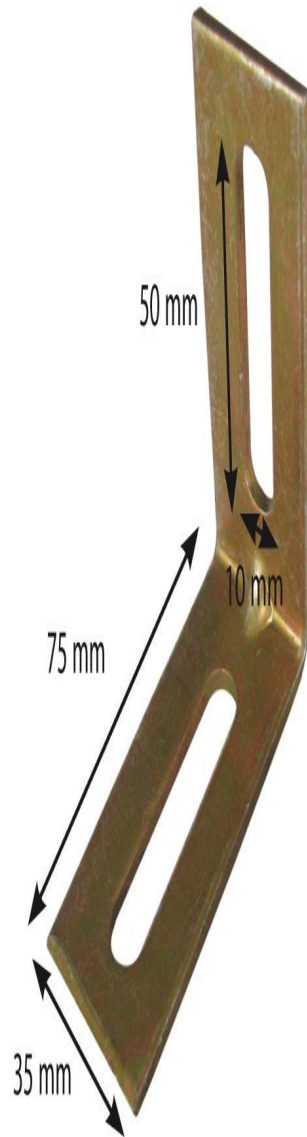
Équerre de marbrier simple
