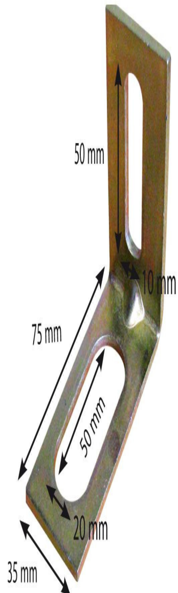
Équerre de marbrier réglable
