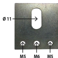
Fixation de rail de volet coulissant ISO à la résine - platine de rail
