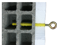
Anneau électricien - vue en coupe
