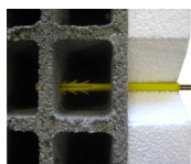
Fixation pour accessoire ISO - vue en coupe
