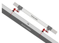
Fixation solaire filet métrique - schéma
