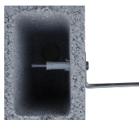
Cheville parpaing - Vue en coupe
