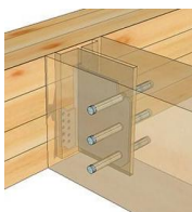
Etrier à âme avec encoche - vue en situation
