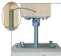
Pied de poteau réglable avec usinage M24 - vue en situation
