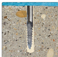
Douille Inox A4 à la résine - vue en coupe
