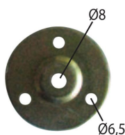
Rosace support main courante avec trous
